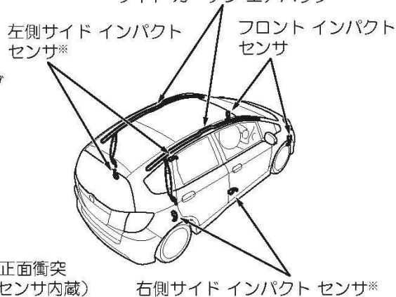
サイド カーテン エアバッグ※
