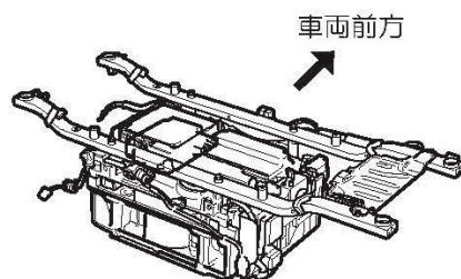
IMA バッテリー（100V）
