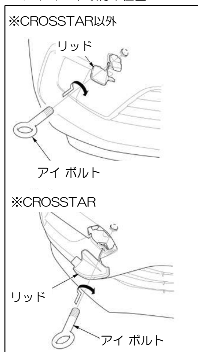
アイ ボルト取付け位置
