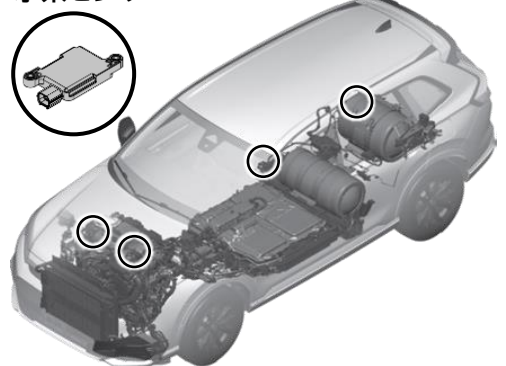
水素センサ
