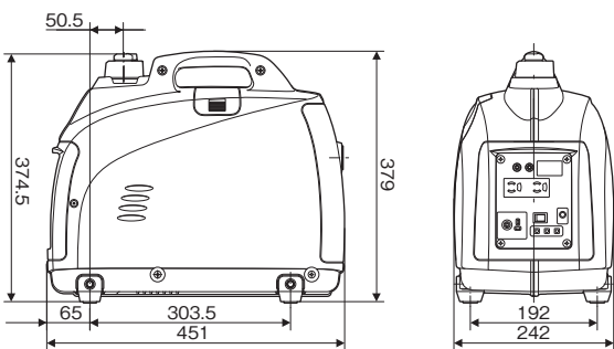
外観寸法図
