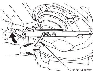
LLAVE DINAMOMETRICA
