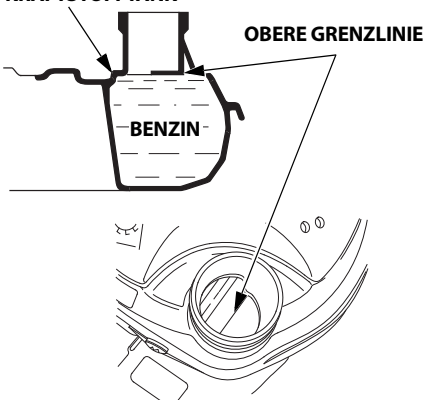
KRAFTSTOFFTANK
