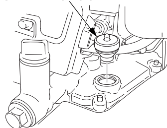
TAPÓN DE LLENADO DE ACEITE DE LA TRANSMISIÓN
