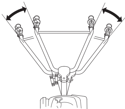
DISPOSITIF DE REGLAGE D'ANGLE DE MANCHERON
