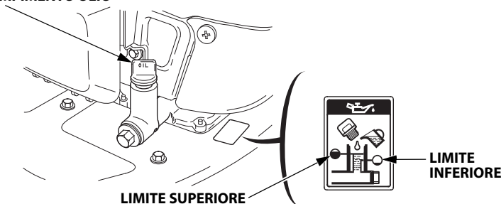
TAPPO DI RIEMPIMENTO OLIO
