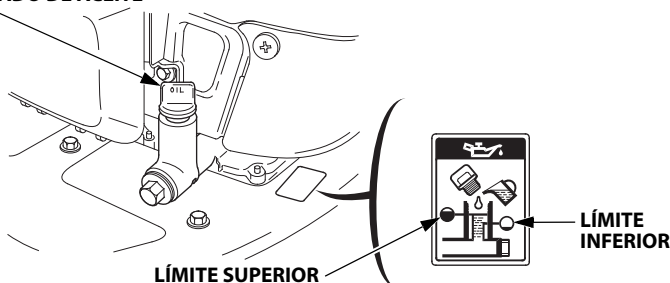
TAPÓN DE LLENADO DE ACEITE
