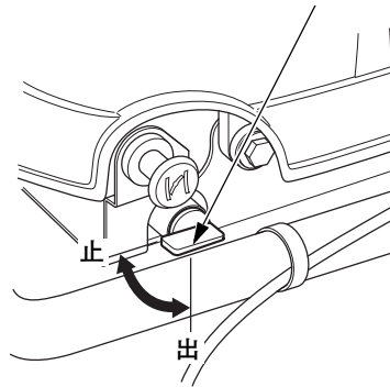
燃料コックレバー
