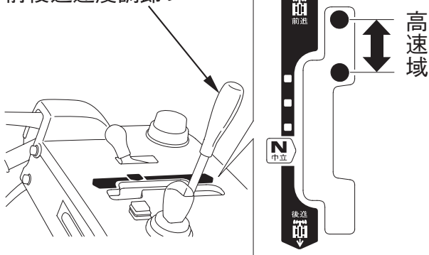
前後進速度調節レバー
