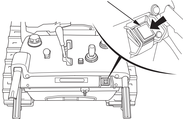
除雪クラッチボタン (表示灯内蔵)
