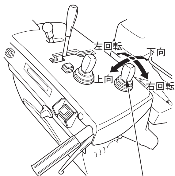
投雪方向調節スイッチ
