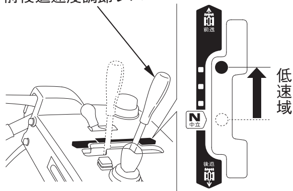
前後進速度調節レバー
