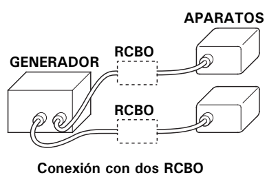
Conexión con dos RCBO
