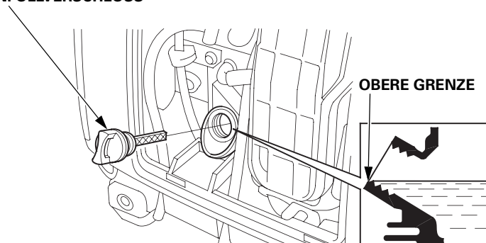
ÖLEINFÜLLVERSCHLUSS
