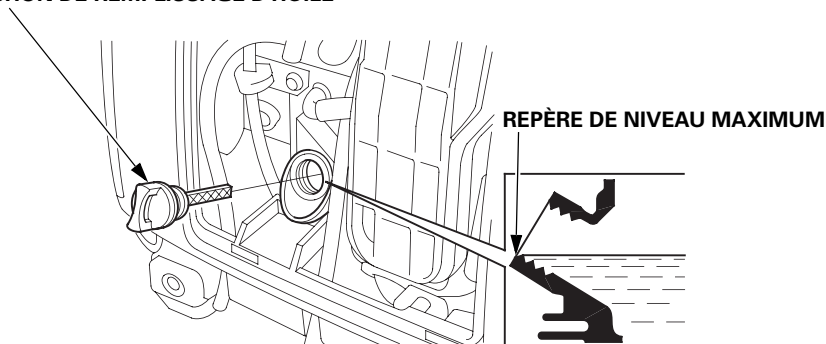
BOUCHON DE REMPLISSAGE D'HUILE
