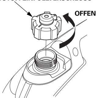
KRAFTSTOFFEINFÜLLVERSCHLUSS
