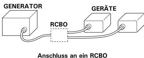
Anschluss an ein RCBO
