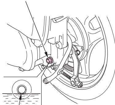
オイルチェックボルト
