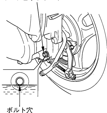
オイルチェックボルト
