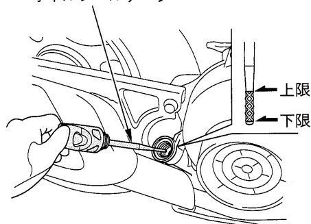
オイルレベルゲージ
