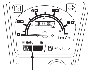
燃料計
