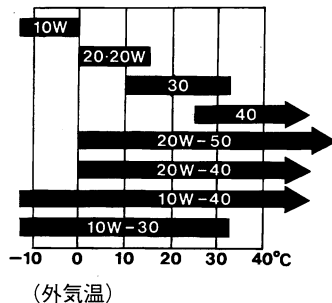
気温と粘度との関係
