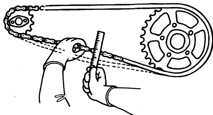
ドライブチェーンのたるみ
