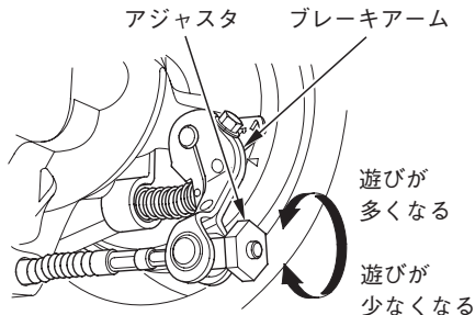
《右側アジャスタ》(左右供)
