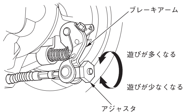
《右側アジャスタ》(左右共)
