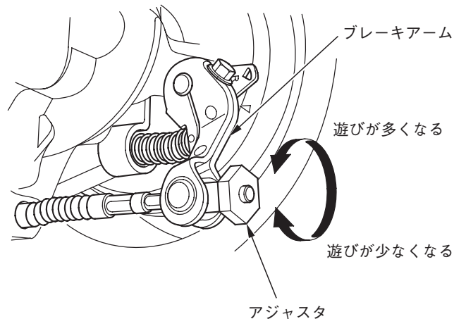
《右側アジャスタ》(左右共)
