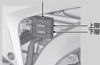
後輪ブレーキリザーバタンク
