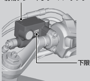
前輪ブレーキリザーバータンク
