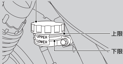
後輪ブレーキリザーバートank
