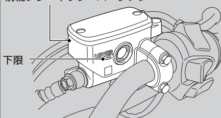
前輪ブレーキリザーバートank
