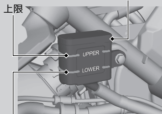
リア 後輪ブレーキリザーバータンク
