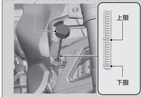
リザーバータンクキャップ／レベルゲージ
