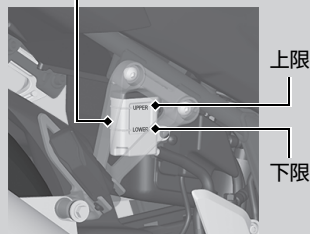
後輪ブレーキリザーバタンク
