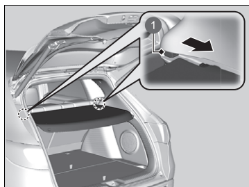
① サポートラッチ
