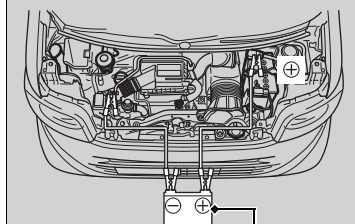
ターボ装備車 救援車のバッテリー
