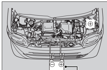
ターボ非装備車 救援車のバッテリー
