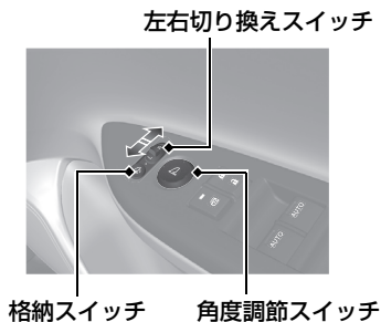
格納スイッチ
