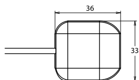
平面図
