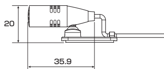
[側面図]
