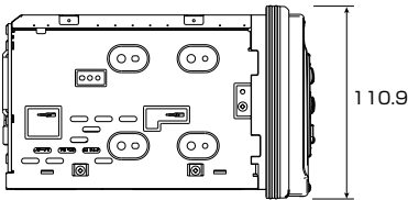
〔左側面図〕
