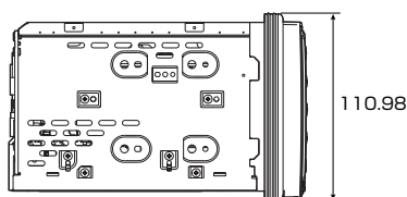
[左側面図]
