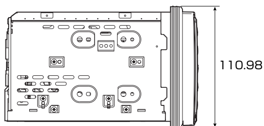
[左側面図]
