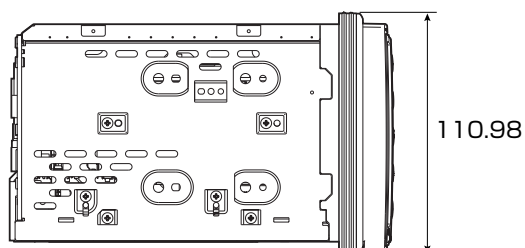
[左側面図]
