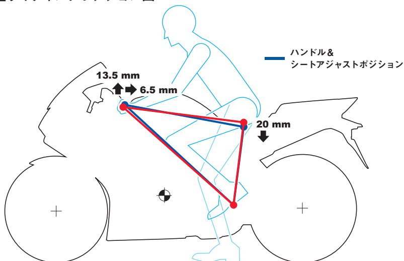
■ライディングポジション図
