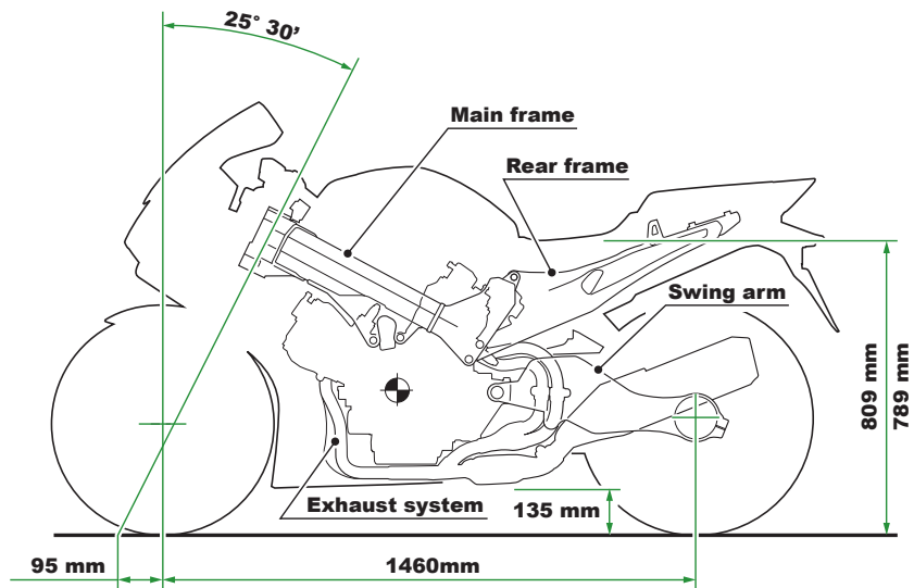
■ディメンション図
