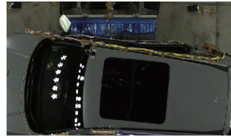
側面衝突
