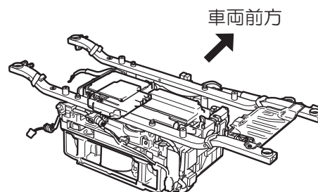
IMA バッテリー（100V）
