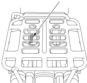
フレーム号機打刻位置
