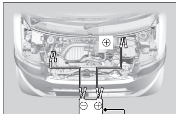
ターボ非装備車 救援車のバッテリー
