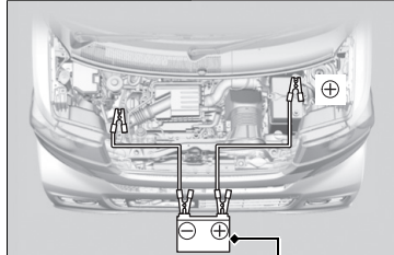
ターボ装備車 救援車のバッテリー
