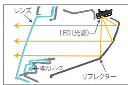
LED光源からリフレクターで反射させ前方に照射
