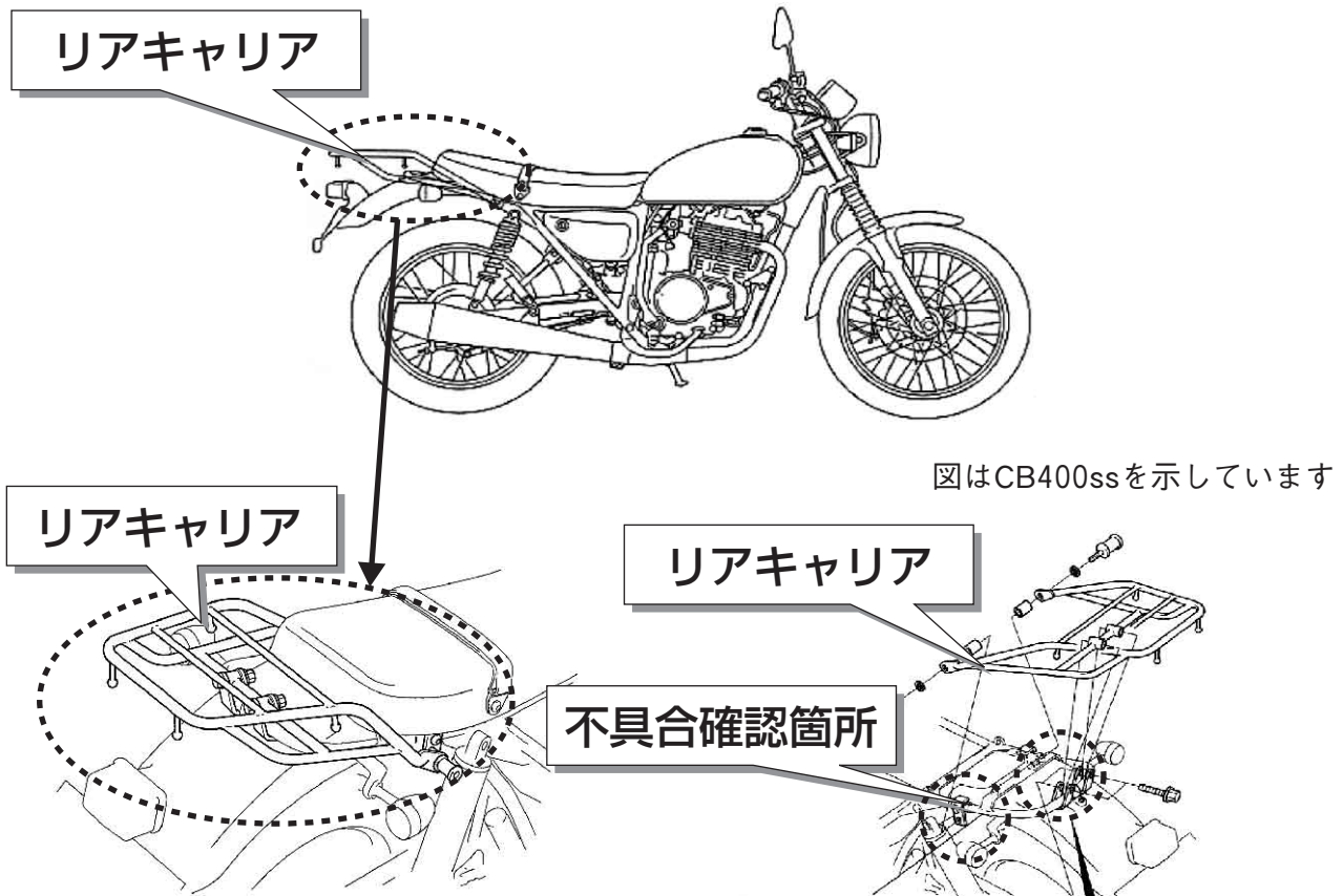
リアキャリア分解図
