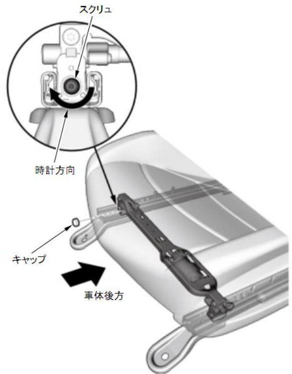
シートを後方へスライドさせる場合
