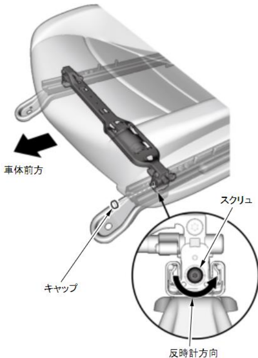
シートを前方へスライドさせる場合
